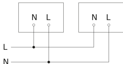
Diagrama electrónico interconexión maestro-maestro
